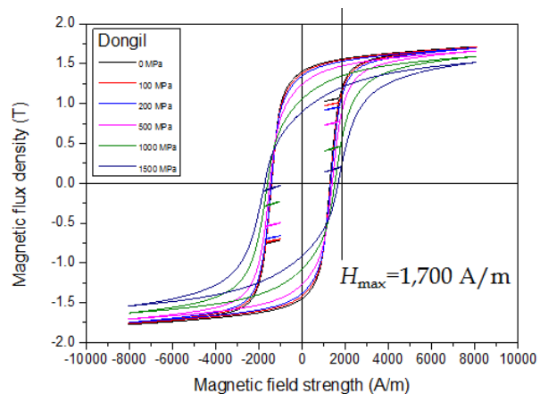
그림 1. 텐던 자기이력곡선 측정 장치 및 텐던(동일제강)의 자기이력곡선
