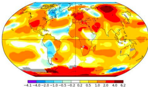
2018년의 지구 표면 온도를 색으로 표현한 그림. 붉을수록 열선이 강함을 뜻한다. / NASA
