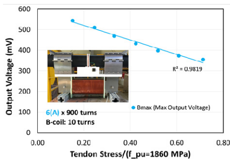
그림 2. 탈부착식 요크와 이를 활용한 텐던의 응력측정 및 단면손상 측정 [3]
