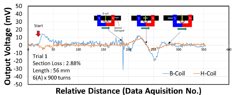
그림 2. 탈부착식 요크와 이를 활용한 텐던의 응력측정 및 단면손상 측정 [3]
