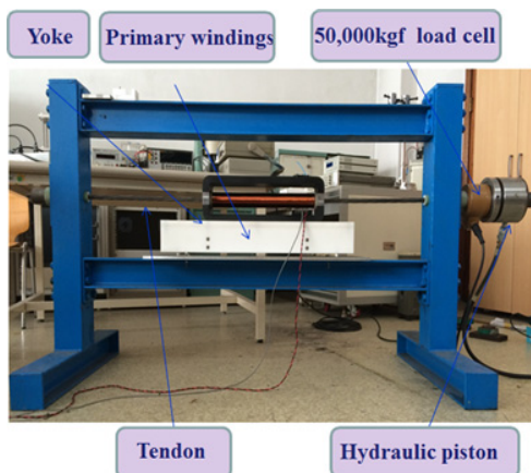
그림 1. 텐던 자기이력곡선 측정 장치 및 텐던(동일제강)의 자기이력곡선
